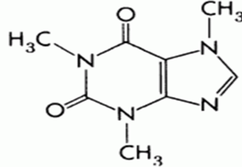
CAFFEINE
